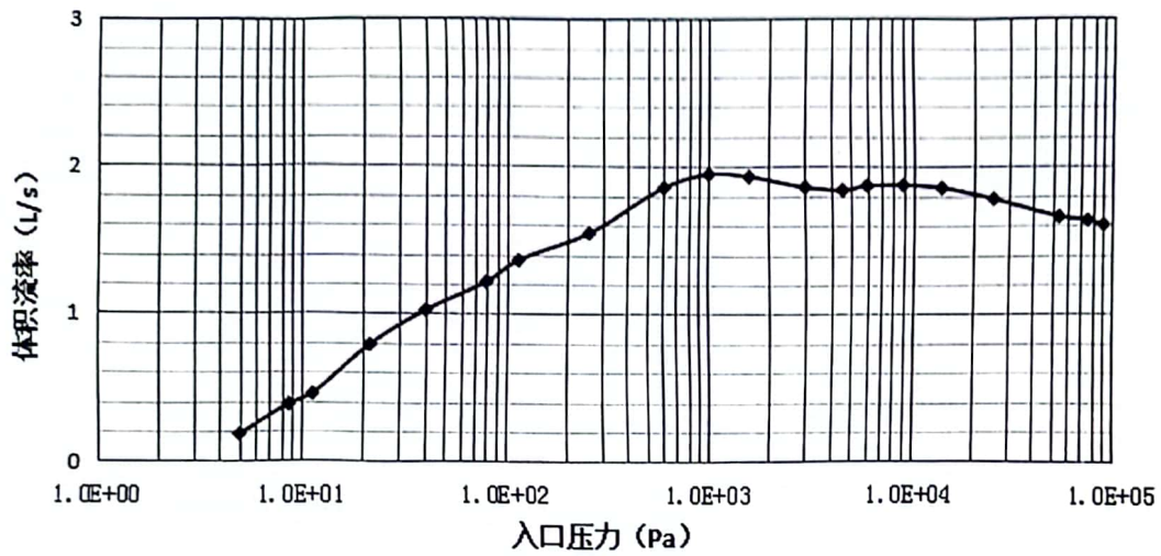
入口压力、体积流率-曲线
