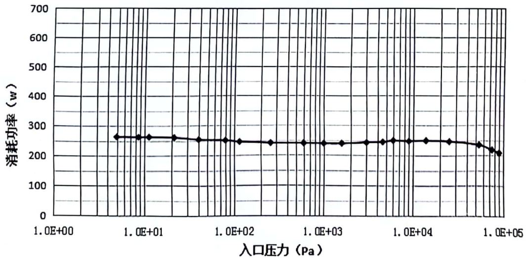
入口压力、消耗功率-曲线
