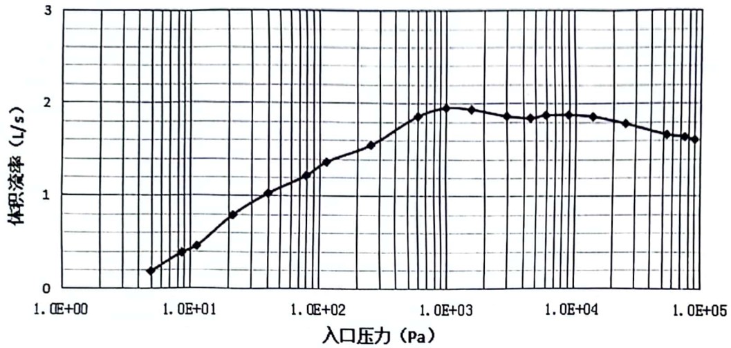
入口压力、体积流率-曲线
